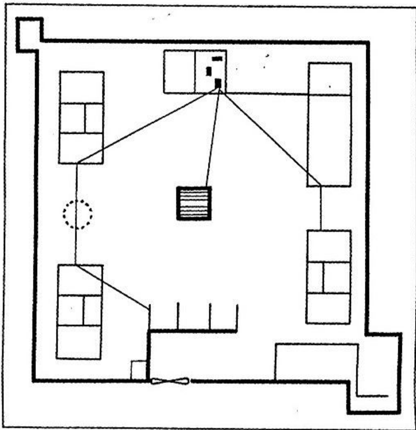
הדגם הסופי של חצר תל-עמל, כפי שתוכנן על-ידי שלמה גור וחבריו. ממדי החצר: 35 x 35 מטר
